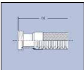
Milchrohr Gewindestutzen DIN 11851
